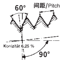
美制NPT锥螺纹
