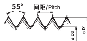
英制G管螺纹 DIN ISO 228
