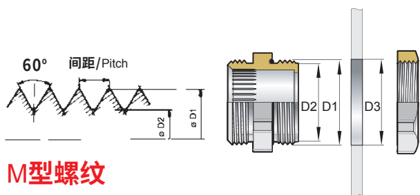
公制ISO螺纹EN60423
