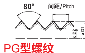
德制PG螺纹 DIN 40430
